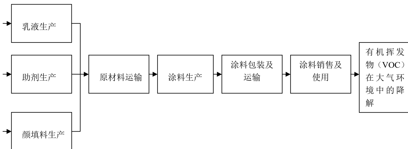
图B.1 水性建筑涂料产品生命周期(LCA)系统边界图
